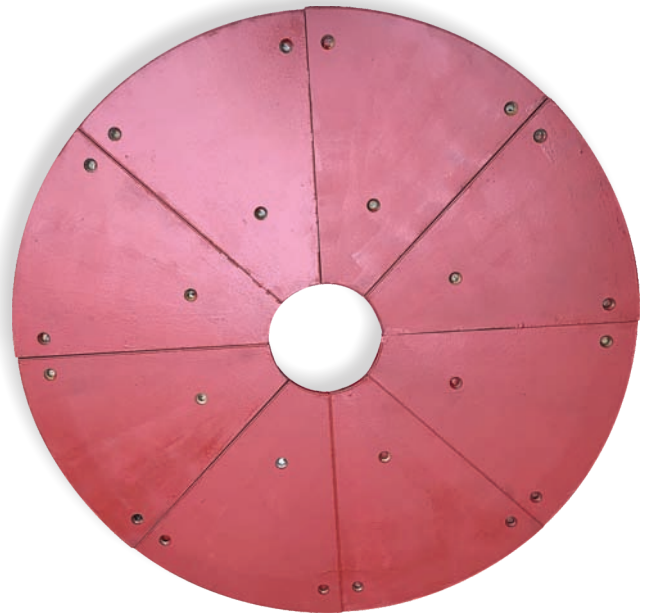
Single Shaft Yan Duvar Aşınma Plakaları
